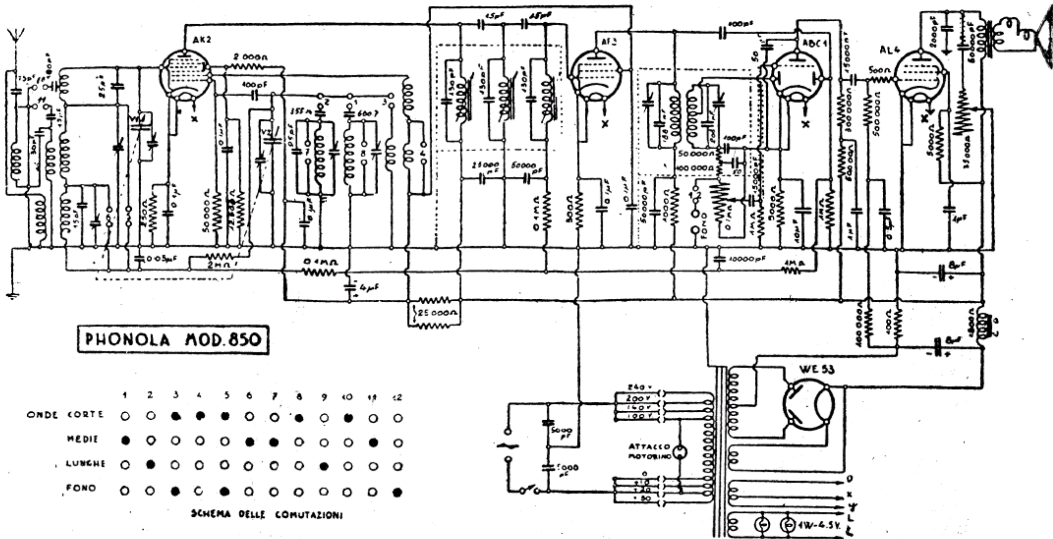
PHONOLA RADIO (S. A. FIMI). — Modelli « 850, 851 e 853 ». - Produzione 1937. - Media frequenza: 470 kHz, (Si vedano i particolari del castello d'alta frequenza nella pagina seguente).
